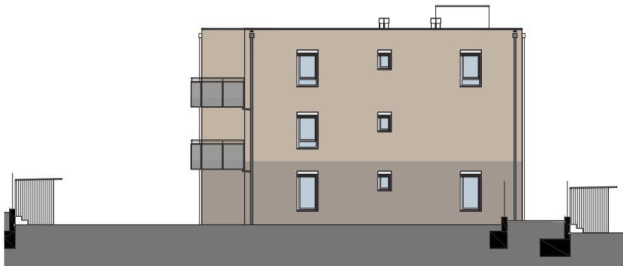
ANSICHT OST
