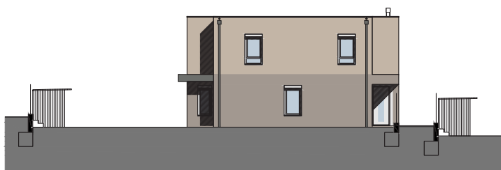
ANSICHT OST
