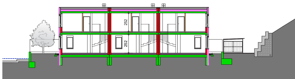
LÄNGSSCHNITT
