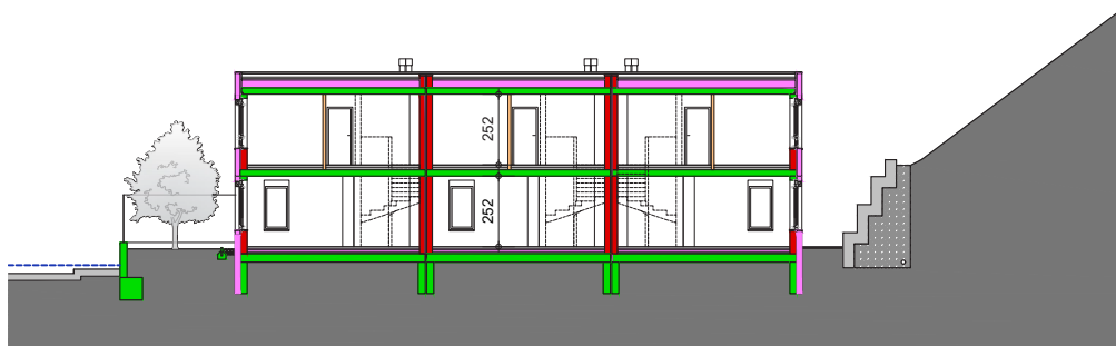
LÄNGSSCHNITT
