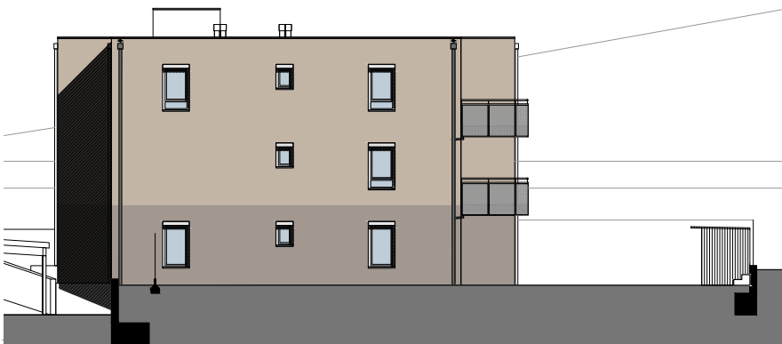
ANSICHT WEST
